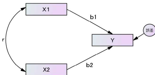
図1.基本的な重回帰分析モデル
