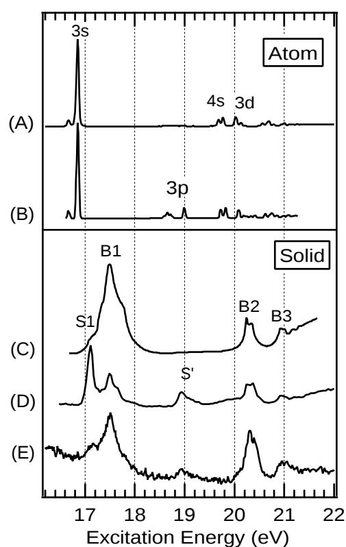
図 1: Ne を標的とした電子的励起状態の生成スペクトル。
